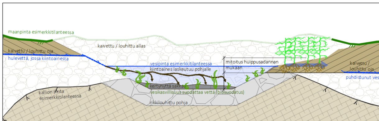
Kuva 10. Periaate kuva alueelle rakennettavista viivytyksistä sekä pajukkosuodatuksista
